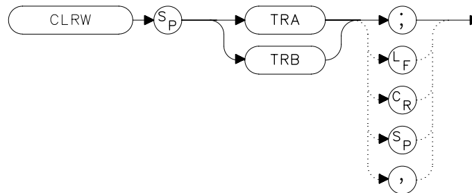
CLRW Syntax
