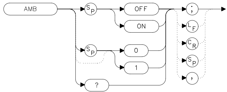
Figure 7-45 AMB Syntax
